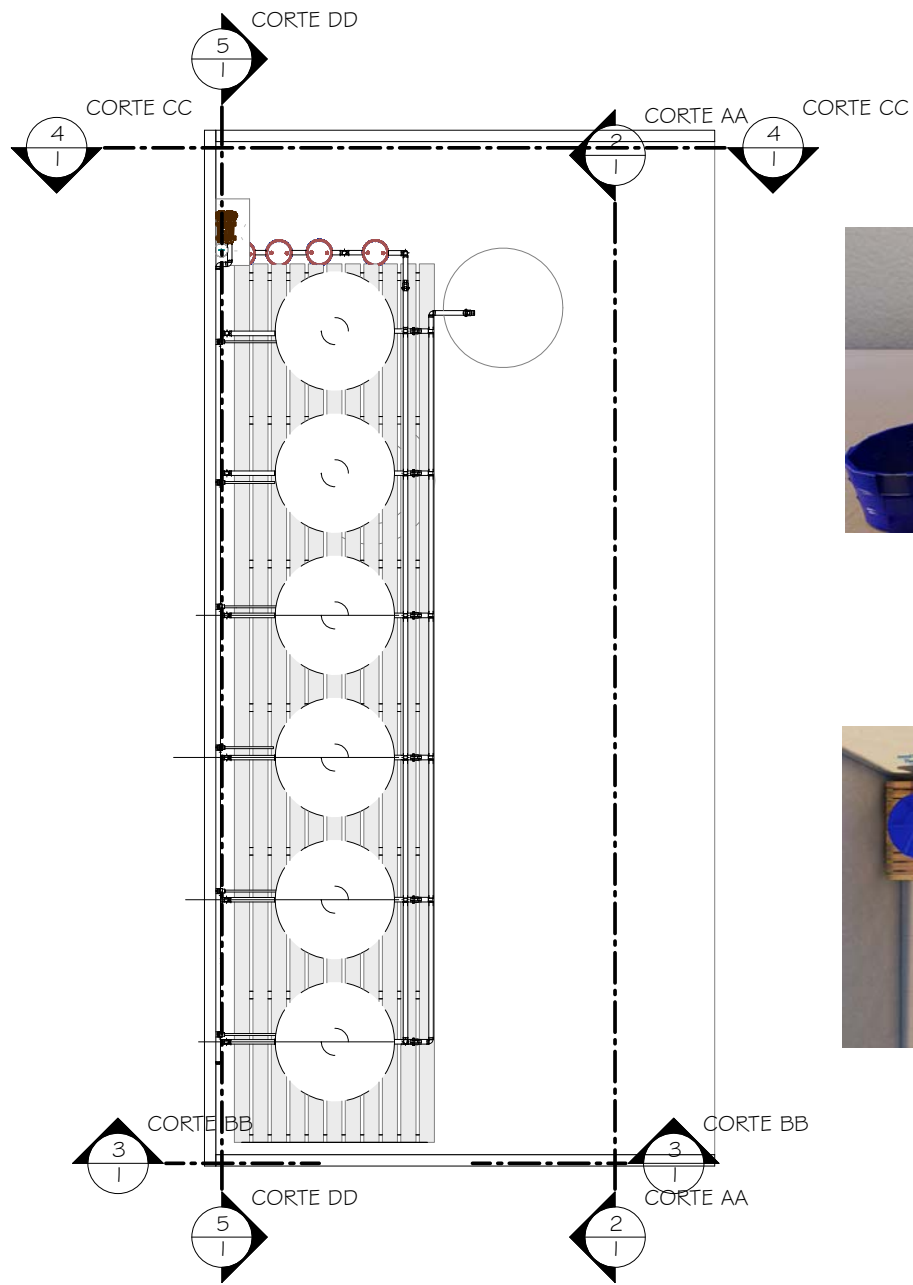
1 Vista Planta Baixa 1 : 100
